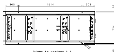
Vista in sezione A-A Scala: 1:15
